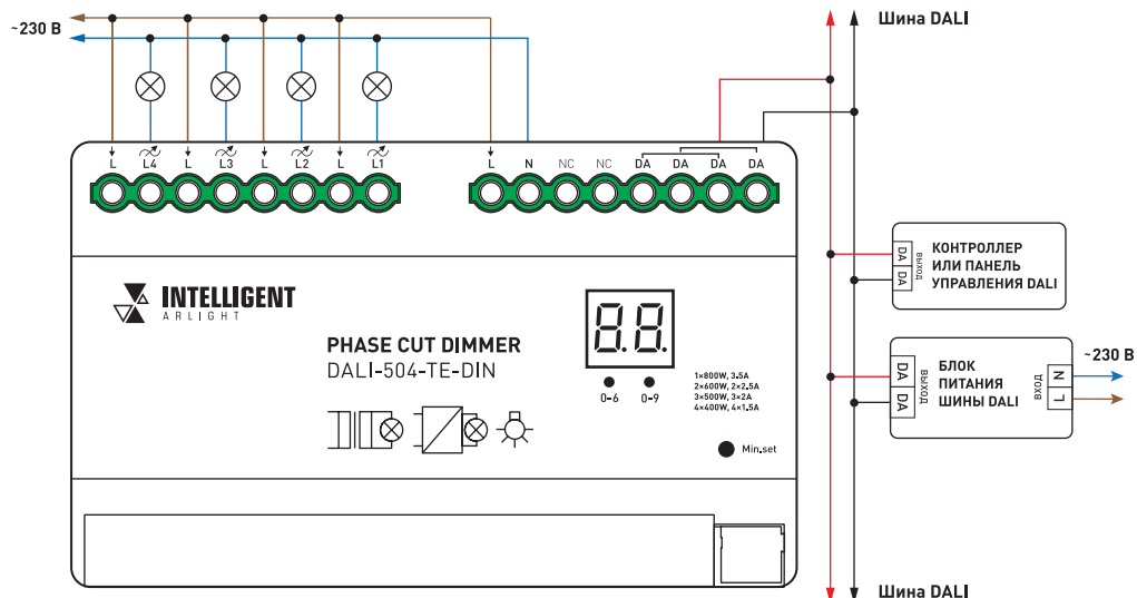
Рисунок 1. Пример схемы подключения диммера DALI-504-TE-DIN.
